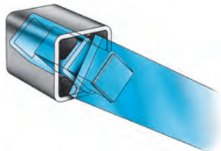
Raccords enfichables : carré intérieur en acier tubulaire, bras de levier avec profil carré soudé
