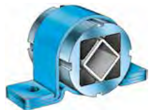
Aussengehäuse mit Befestigungsbride BK
